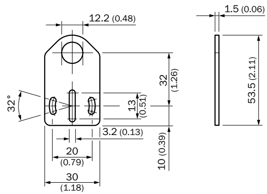
BEF-WG-M12(N)
